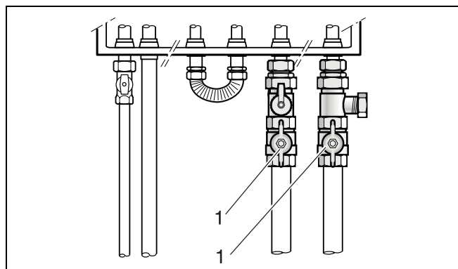
Fig. 5 Rubinetti di manutenzione
